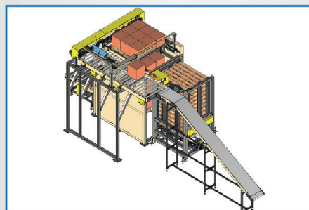
MÁY XẾP PALLET TỐC ĐỘ CAO
