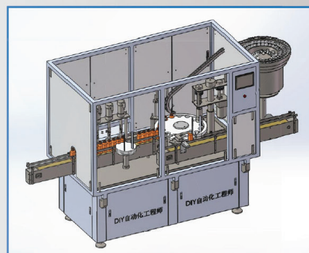
MÁY CẤP LINH KIỆN VÀ LẮP RÁP
