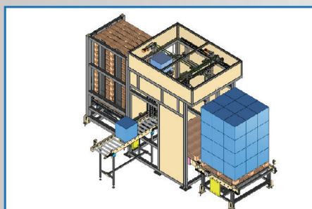
MÁY XẾP PALLET 3 TRỤC
