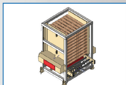
MÁY CẤP PALLET TỰ ĐỘNG
