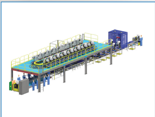
DÂY CHUYỀN LẮP RÁP
