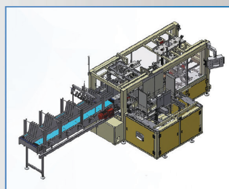
HỆ THỐNG HỖ TRỢ GẮP VÀ CẤP LINH KIỆN
